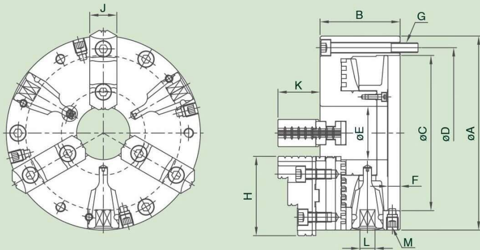
尺寸圖 » Dimensions
