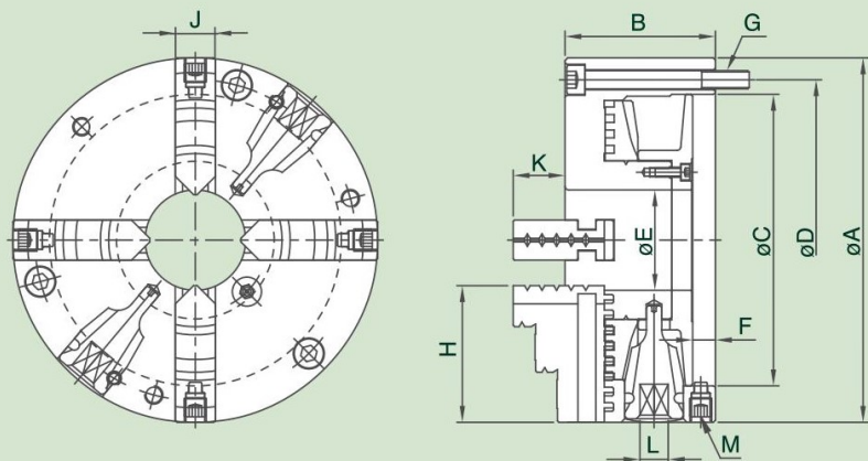
尺寸圖 » Dimensions
