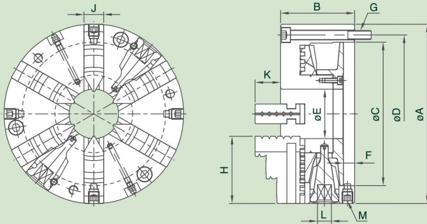
尺寸圖 » Dimensions
